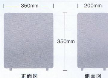
正面図
